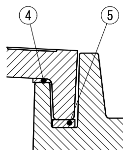
P部拡大図 (1/2)
